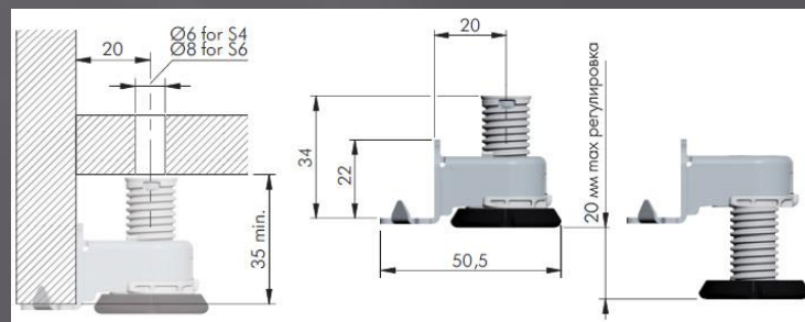
Размеры для опоры с регулировкой 20мм (A и G)
