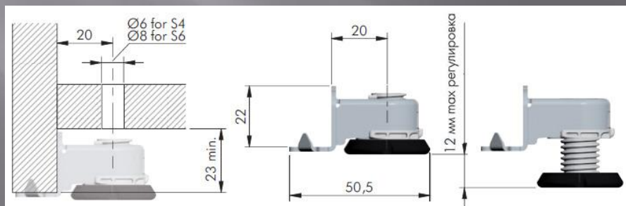
Размеры для опоры с регулировкой 12мм (A и G)
