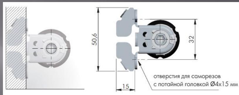
Присадочная карта для опор TECH G
