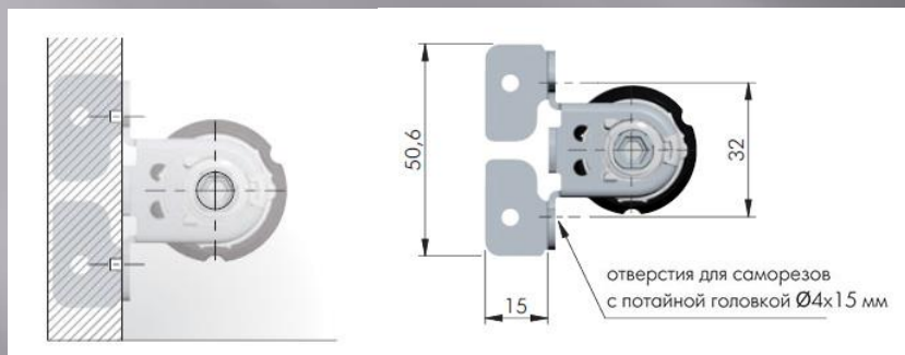
Присадочная карта для опор TECH A
